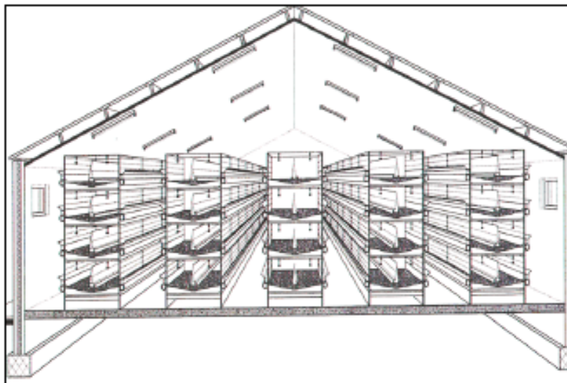
Фиг.3.2а Система за отглеждане в уголемени клетки
