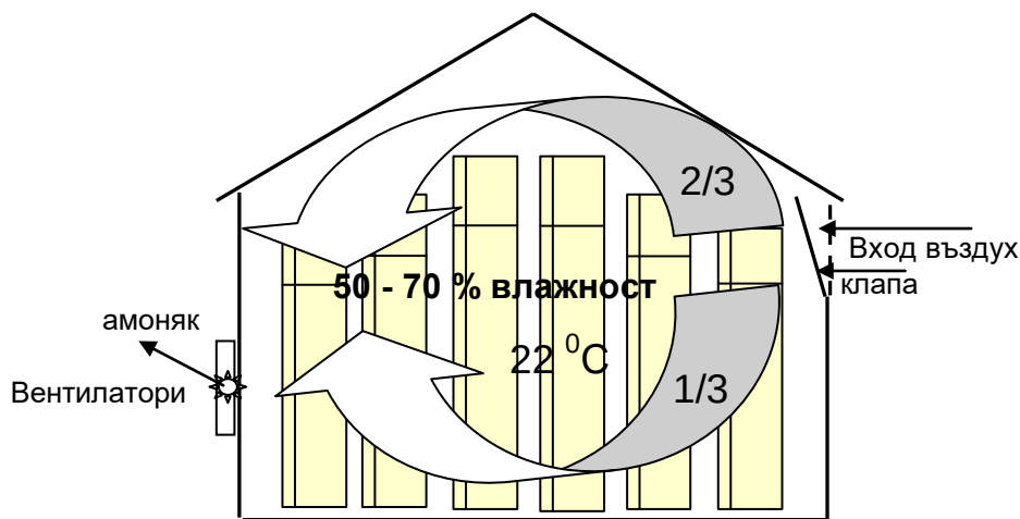
Фиг.3.4 Схема на напречна вентилация
